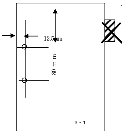
図3 見出し (タブ)
